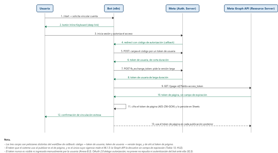
Figura 1. Diagrama de secuencia — vinculación OAuth 2.0.
